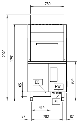
Alzado
